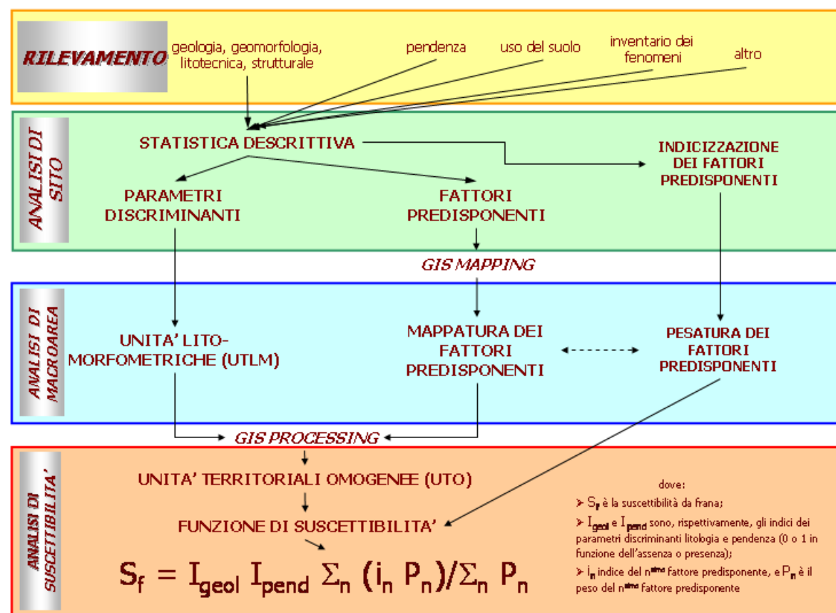
Fig. 1 – Diagramma di flusso illustrante la Metodologia ENEA-Roma Tre
