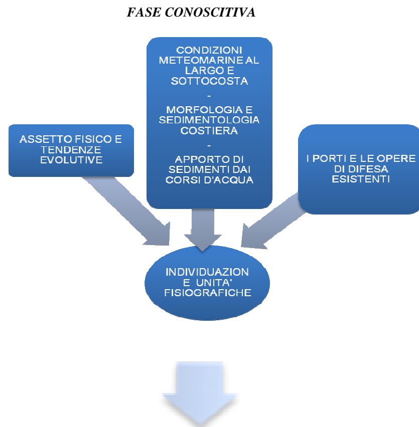
Schema metodologico per l'individuazione delle aree soggette a erosione costiera
